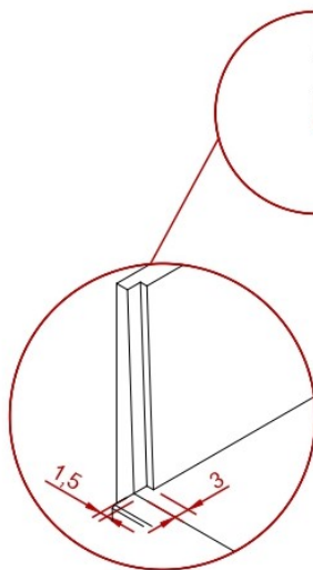
DETALLE A: REBAJE PARA ALOJAMIENTO DE LA TAPA FRONTAL
